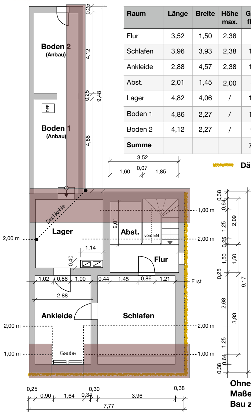
Raumbuch (Innenmasse in m)
